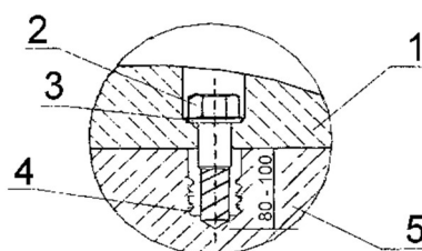
Szczegół A
