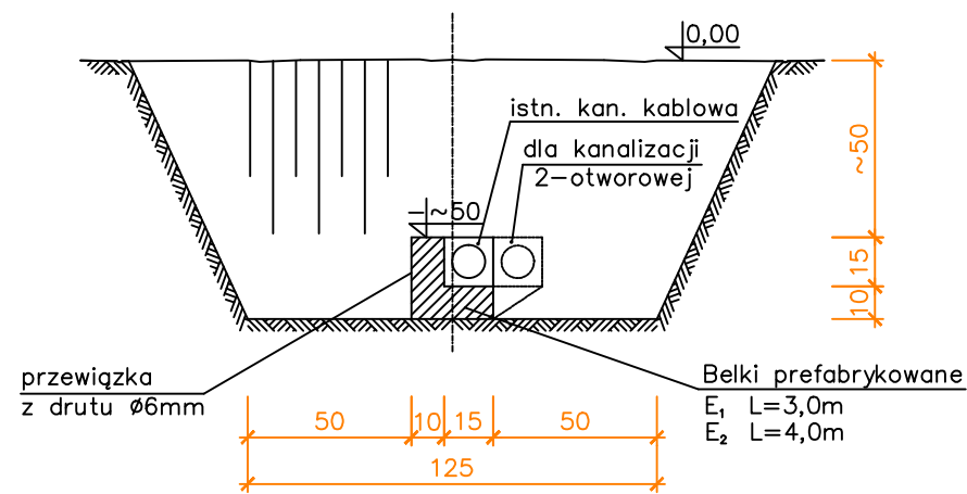
PRZEKRÓJ A-A SKALA 1:25
