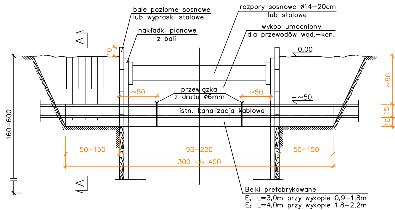
PRZEKRÓJ PODŁUŻNY SKALA 1:25
